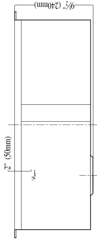
SECTION A-A
